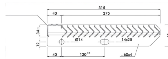
Găurire placă conform UNI 11002-2
