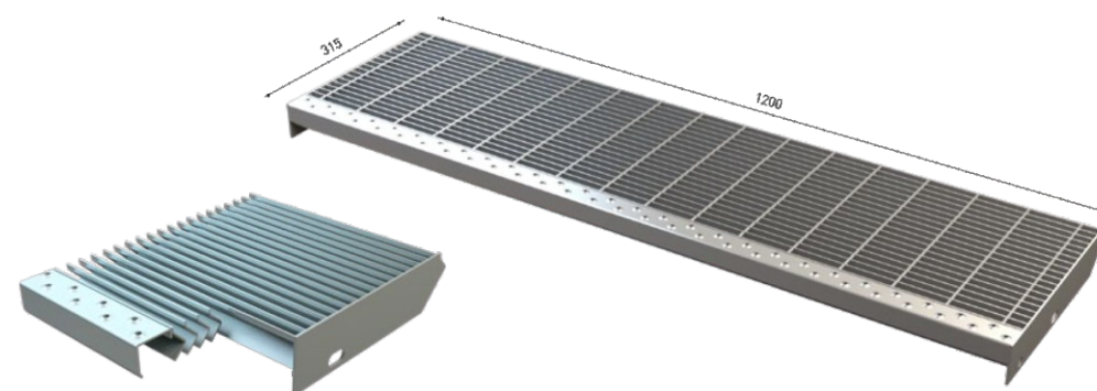
Găurire placă conform UNI 11002-2
