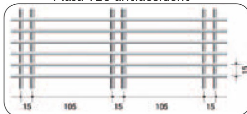
Plasă RT antiaccident
